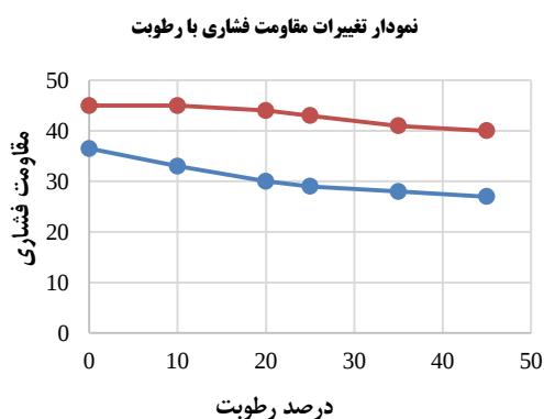
شکل (۹). رابطه مقاومت فشاری تک‌محوره با رطوبت
