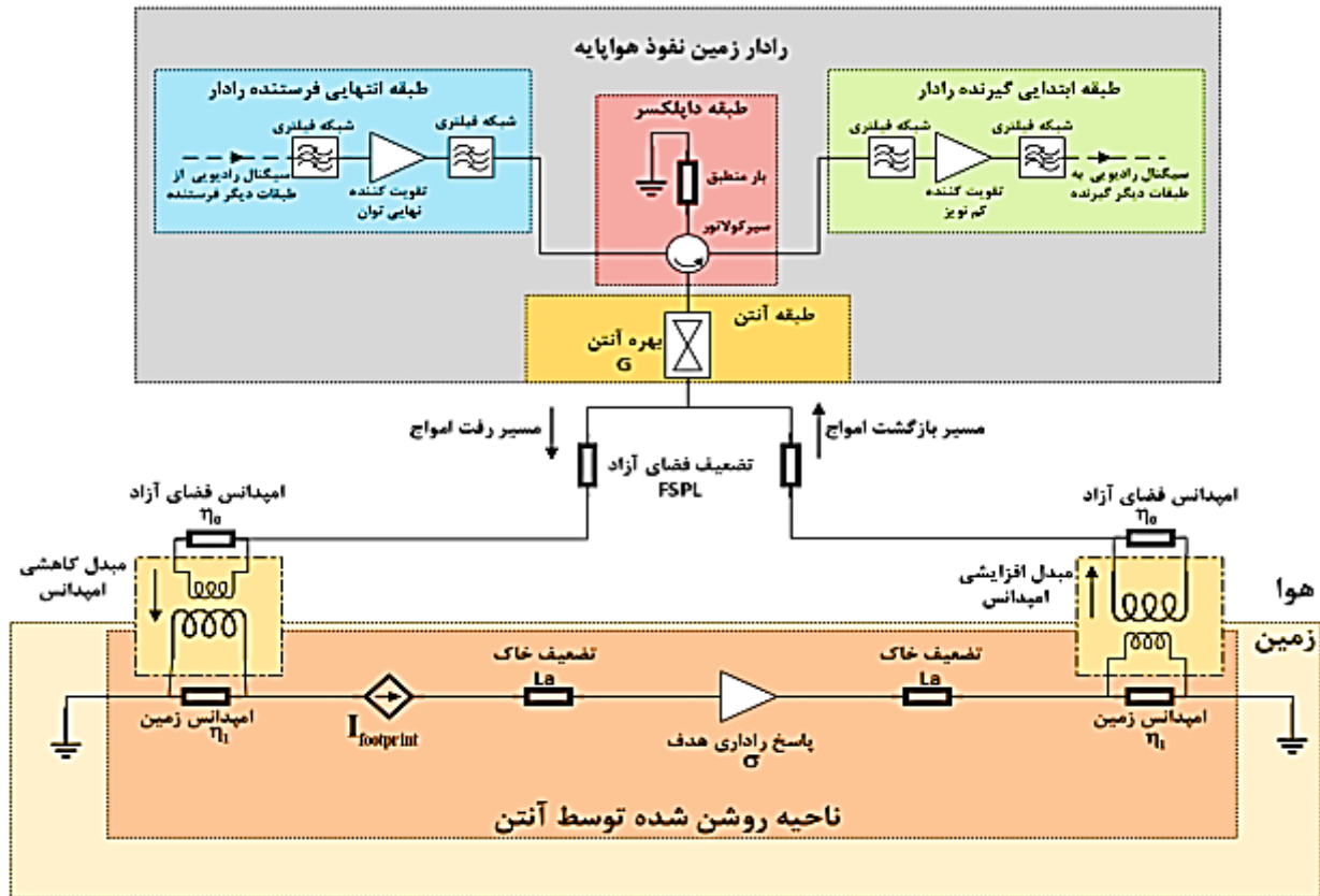
شکل (۲). مدل‌سازی انتشاری یک رادار زمین نفوذ هوا پایه ایستا و نمایش پارامترهای اساسی در فرآیند آشکارسازی هدف مدفون
