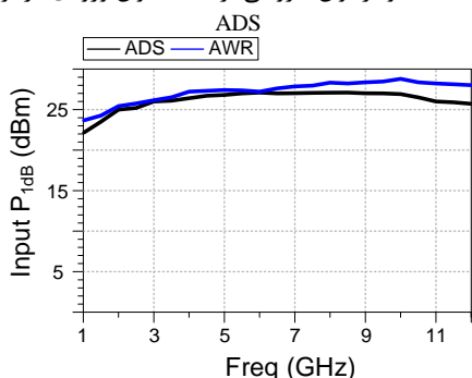
شکل (۱۱). نمودار P_{1dB} ورودی در فرکانس‌های مختلف در دو نرم‌افزار AWR و ADS
