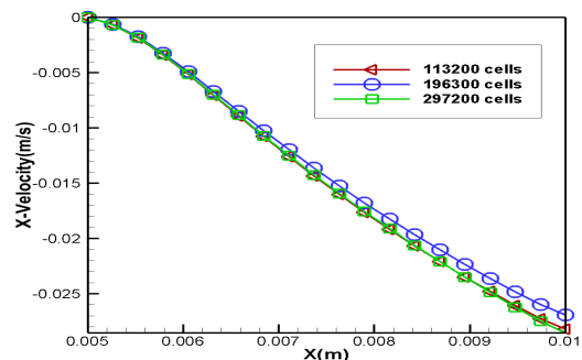
شکل (۴): نمودار مؤلفه افقی سرعت برحسب فاصله افقی در حالت با حضور کنترل کننده
