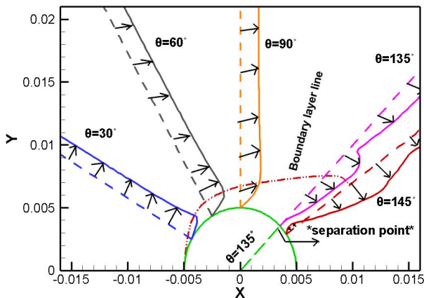
شکل (۱۳): نمودار پروفیل‌های سرعت و لایه‌مرزی بر روی استوانه‌ی با کنترل‌کننده در فاصله X=0/008 \text{ m}
