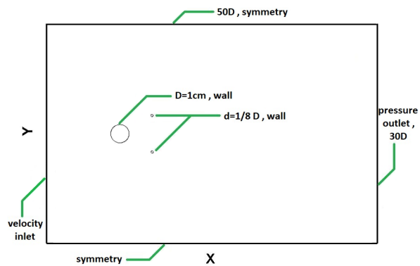
شکل (۱): طرحواره ابعاد کانال و شرایط مرزی
