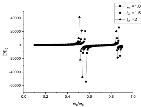
شکل (۵). مطالعه پارامتریک میدان الکتریکی برحسب بسامد
