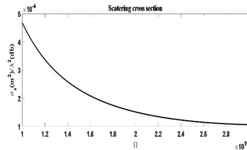
شکل (۱۴). تغییرات سطح مقطع پراکندگی نسبت به بسامد سیکلوترونی
