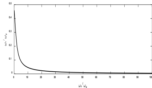
شکل (۱۳). تغییرات بسامد تشدید بهنجار شده بسامد پلاسمایی بر حسب بسامد سیکلوترونی بهنجار شده بسامد پلاسمایی
