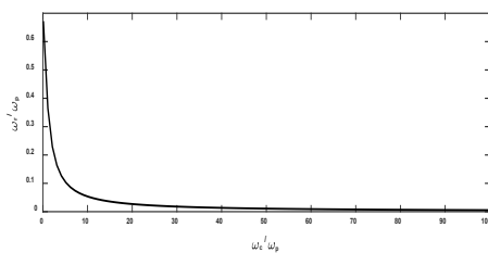
شکل (۶). نمودار تغییرات بسامد تشدید بهنجار شده برحسب بسامد
