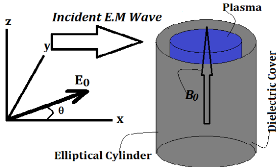
شکل (۲). ستون پلاسمای مغناطیده با سطح مقطع بیضوی با لایه دی الکتریک
