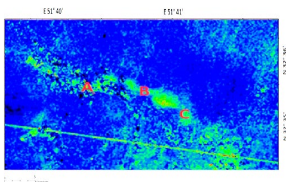
شکل (۱۵). میزان فرونشست در گذر پیکسل‌های مجاور حفر تونل
