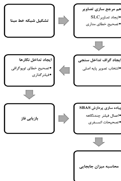
شکل (۷). فلوچارت الگوریتم تداخل‌سنجی
