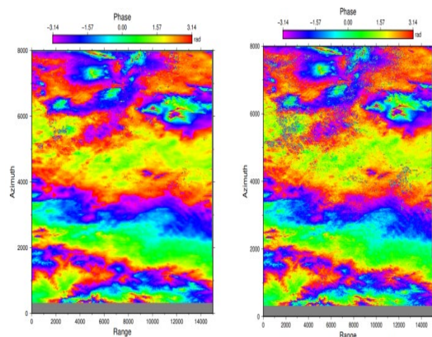
شکل (۱۰). اعمال فیلتر گلدستاین بر روی تداخل نماهای سری زمانی
