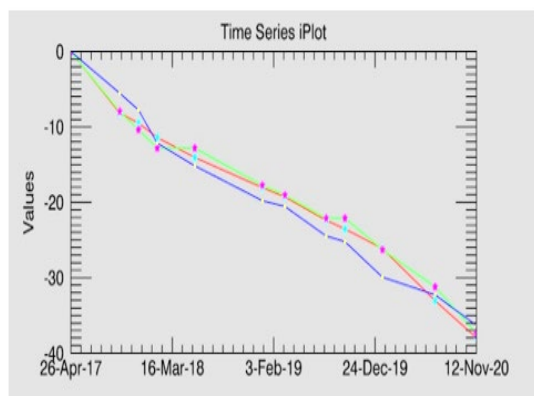
شکل (۱۶): میزان فرونشست پیکسل‌های فوقانی هدف برحسب (mm/year)
