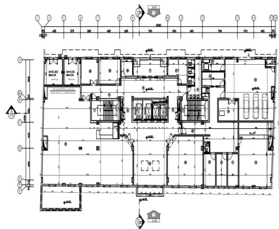
شکل (۵): پلان همکف سازه مطالعه موردی
