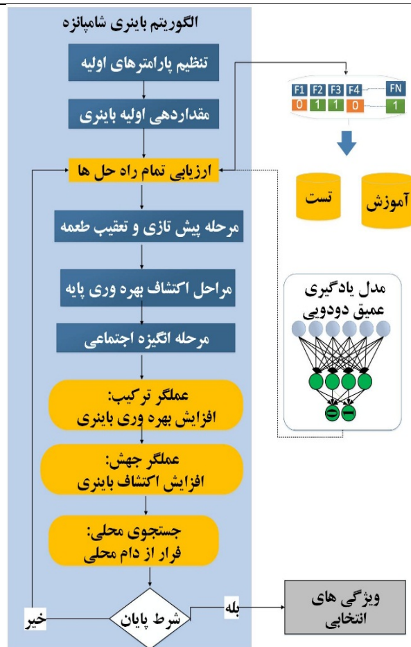
شکل (۲): فلوچارت روش پیشنهادی انتخاب ویژگی BCHO
