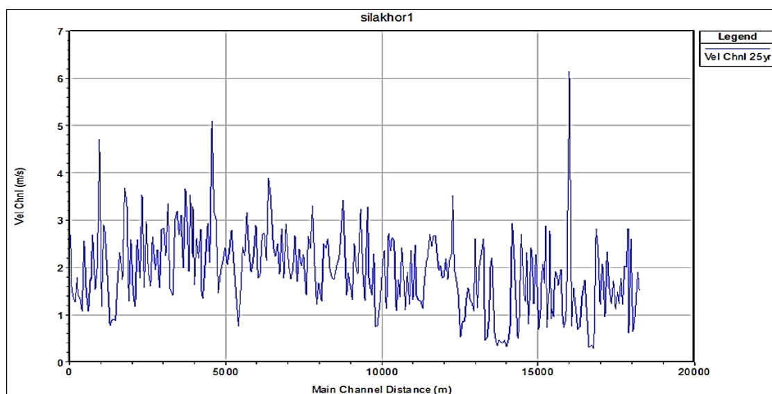
شکل (۷). نمودار تغییرات سرعت جریان در طی رودخانه سیلاخور ۱ در شرایط موجود به ازای سیل ۲۵ ساله
