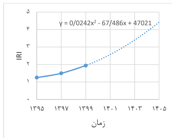
شکل (۱۰). منحنی تغییرات ده‌ساله پیش‌بینی شده شاخص IRI آزادراه قم - گرمسار
