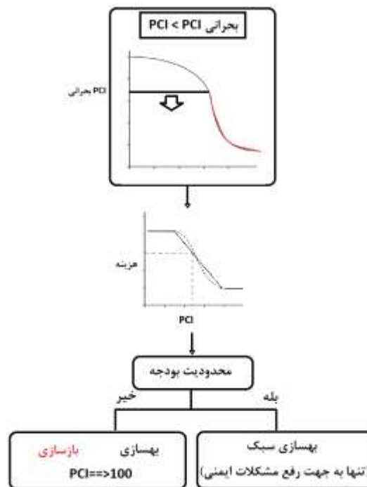
شکل (۷). فلوچارت برنامه تعمیر و نگهداری برای حالت پس از شرایط بحرانی خرابی
