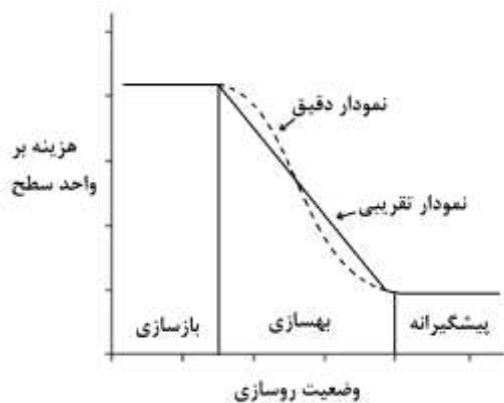
شکل (۴). مقدار هزینه در واحد سطح روسازی به ازای شرایط روسازی [۲]
