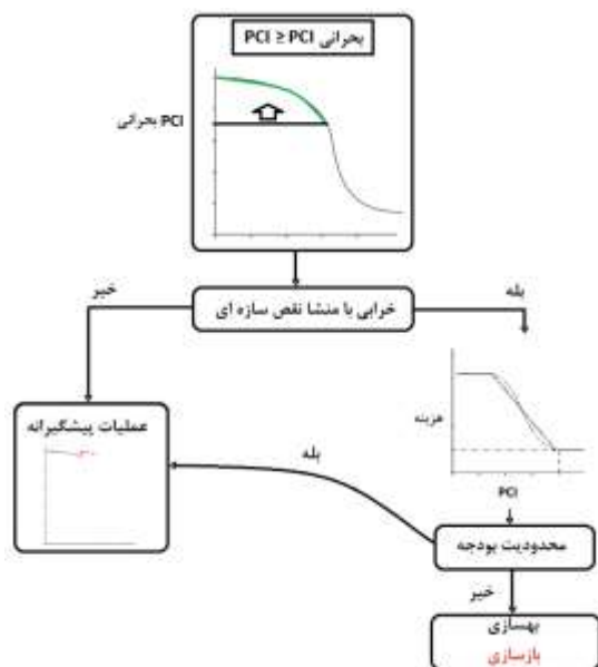
شکل (۶). فلوچارت برنامه تعمیر و نگهداری برای حالت پیش از شرایط بحرانی خرابی
