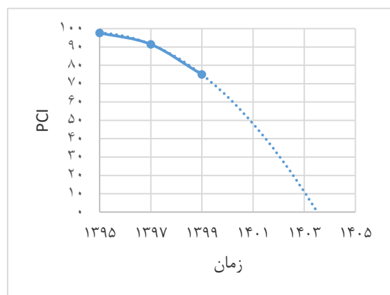
شکل (۱). نمودار پیش‌بینی تغییرات ده‌ساله شاخص PCI آزادراه‌های کشور
