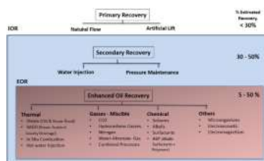
شکل (۴). مراحل برداشت از میدان‌های نفتی
