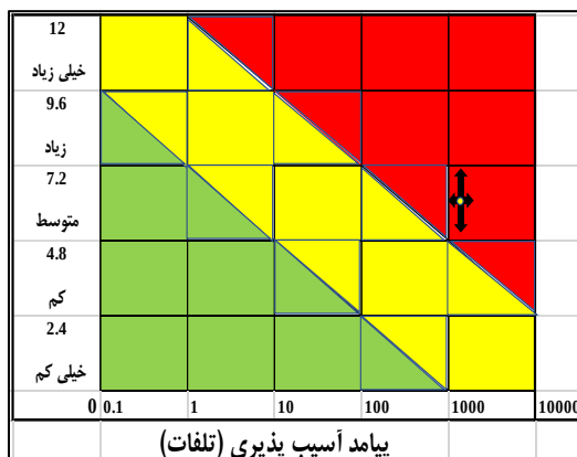
شکل (۱۸). ماتریس تلفات ناشی از ریزش توده های اسلیتی
