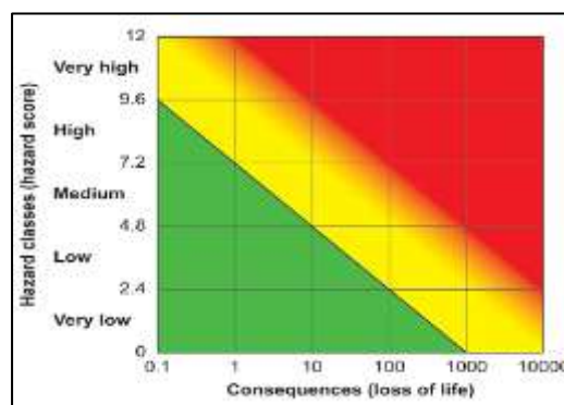
شکل (۱۳). ماتریس خطر ریزش (ری نالد ۲۰۱۲)
