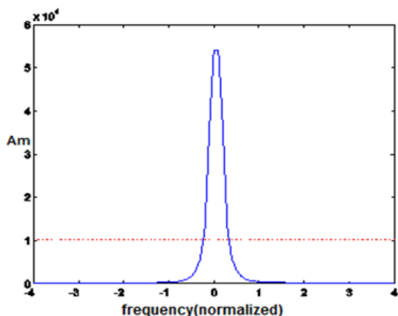
شکل ۷. هیستوگرام فرکانس لحظه‌ای سیگنال ۸-QAM بر حسب دامنه
