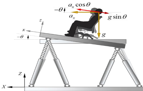
شکل (۴): تصویر مفهومی از حرکت همانگ زاویه ای در مانور شیب- انتقالی
