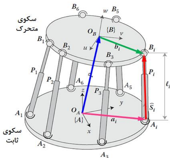
شکل (۱): سکوی استوارت همراه با چارچوب الصاق شده بر سکوی ثابت و متحرک [۱۵]
