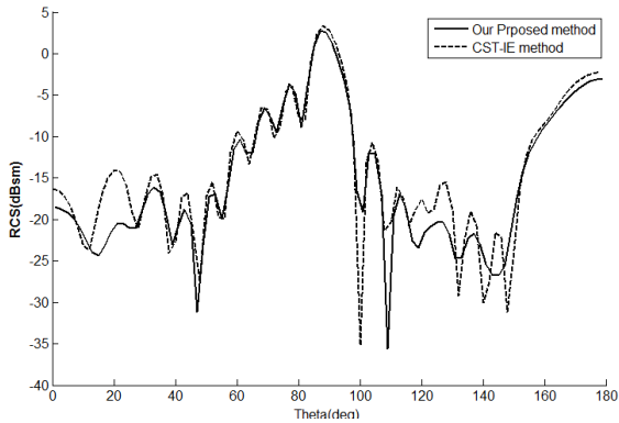
شکل ۱۴. RCS شکل ۹ (عایق) در فرکانس ۶۰۰ MHz برای قطبش موازی
