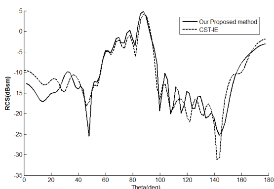
شکل ۲۰. RCS شکل ۱۸ (ترکیب عایق- هادی) در فرکانس ۶۰۰ MHz برای قطبش عمودی
