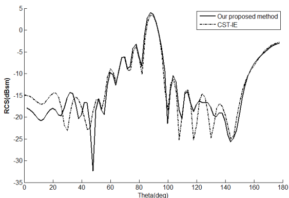
شکل ۱۶. RCS شکل ۱۵ (عایق-ترکیبی) در فرکانس ۶۰۰ MHz برای قطبش عمودی
