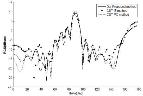
شکل ۱۲. RCS شکل ۹ در فرکانس ۶۰۰ MHz برای قطبش عمودی
