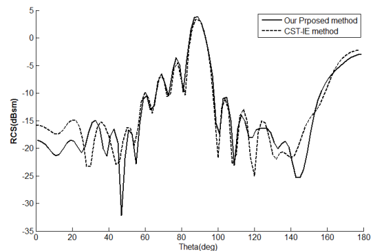
شکل ۱۳. RCS شکل ۹ (عایق) در فرکانس ۶۰۰ MHz برای قطبش عمودی
