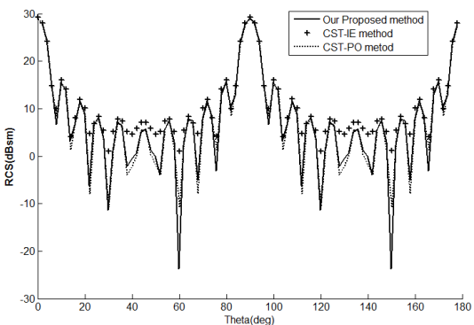
شکل ۶. RCS شکل ۴ در فرکانس ۶۰۰ MHz برای قطبش عمودی
