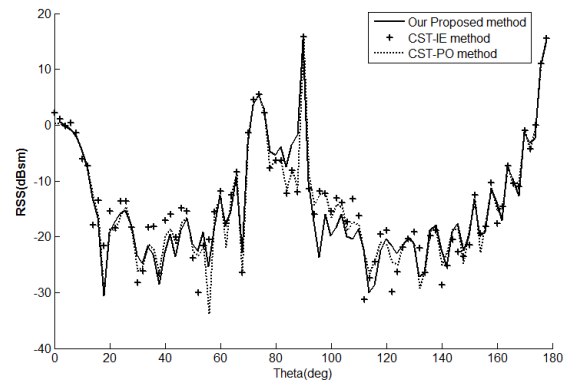
شکل ۲۱. RCS در فرکانس ۳ GHz برای قطبش موازی
