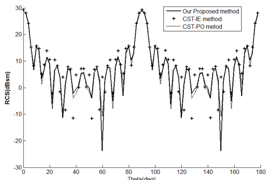
شکل ۵. RCS شکل ۱۰ در فرکانس ۶۰۰ MHz برای قطبش موازی
