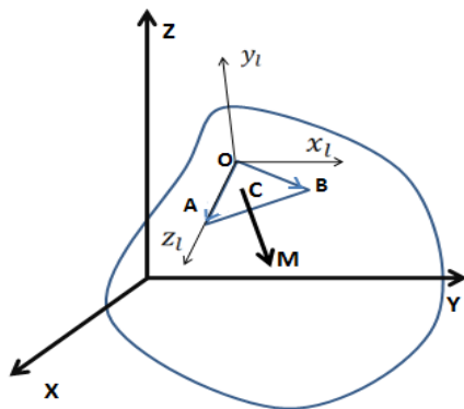
شکل ۱. نحوه مش‌بندی و یافتن بردار عمود بر هر مش
