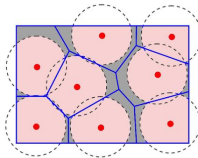
شکل (۸): استفاده از دیاگرام ورونوی برای کشف حفره‌های پوششی (مناطق سایه) در یک شبکه رادار
