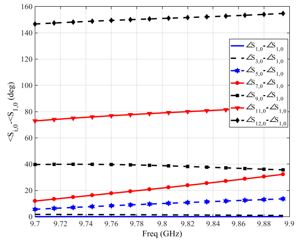
شکل (۱۵): نمودار \langle S_{i,0} - S_{1,0} \rangle_{deg} شبکه تغذیه آنتن به ازای i = 1, 3, 5, 7, 9, 11, 12
