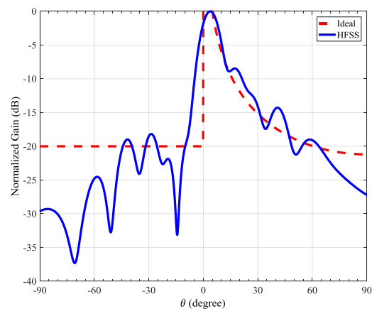
شکل (۱۹): مقایسه الگوی تشعشی آنتن در نرم‌افزار HFSS و حالت ایده‌آل در فرکانس ۹/۸ GHz
