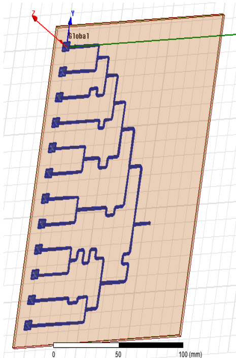
شکل (۱۷): ساختار کامل آرایه خطی میکرواستریپ ۱۲×۱
