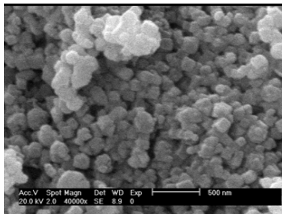
شکل ۱. تصویر SEM مربوط به نانو \text{Fe}_3\text{O}_4
