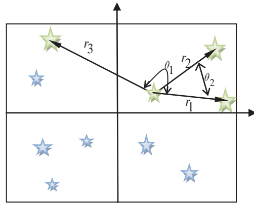
شکل ۳. تشکیل بردار طرح در روش شبکه عصبی [۱۵]
