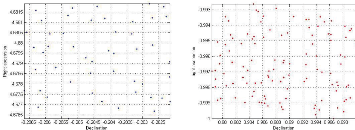
شکل ۱۰. ستارگان استخراج شده از کاتالوگ در اپک مشاهداتی بر حسب رادیان. سمت چپ داده‌های اول، سمت راست داده‌های دوم
