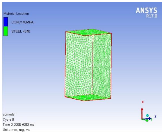
شکل ۲. پلایت فولادی به ضخامت ۲ سانتی‌متر با تقارن یک‌چهارم که جایگزین شبکه میل‌گرد شده است
