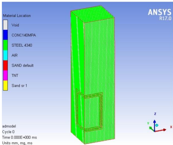
شکل ۳. محیط اوپلری حاوی خاک، هوا و TNT با تقارن یک‌چهارم و مش‌بندی آن
