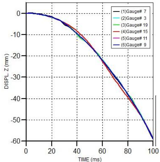
شکل ۱۰. نمودار زمان- جابجایی در راستای z گنج‌های نود سازه
