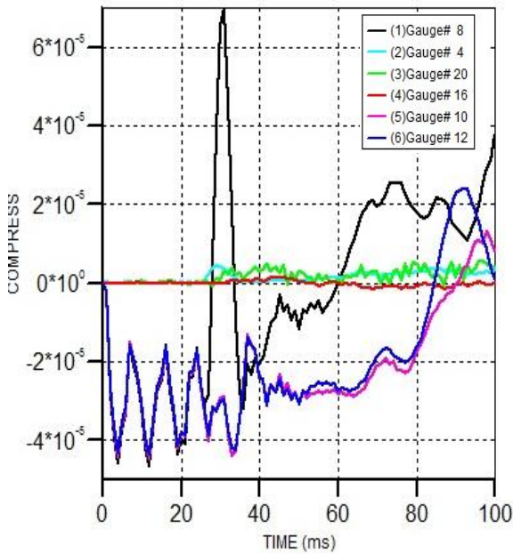
شکل ۱۲. نمودار زمان- فشردگی گنج‌های المان سازه
