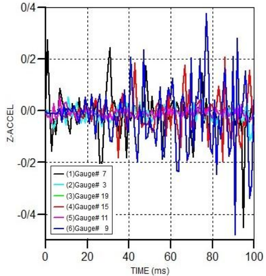
شکل ۹. نمودار زمان - شتاب در راستای z گنج‌های نود سازه
