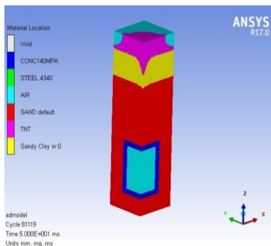
شکل ۱۳. وضعیت پایان تحلیل برای حالت اول
