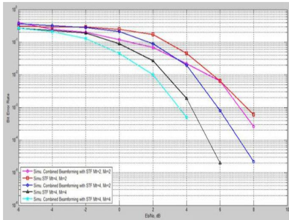
شکل ۱۱. عملکرد نرخ خطای بیت برای روش‌های مختلف به ازای تعداد آنتن‌های فرستنده و گیرنده متفاوت
