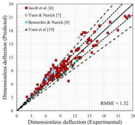
شکل (۱۲): مقایسه بین پیش‌بینی مدل تجربی ارائه‌شده در معادله ۶ [۱۰] و مقادیر تجربی برای بارگذاری محلی
