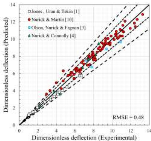
شکل (۹): مقایسه بین پیش‌بینی مدل تجربی ارائه‌شده در معادله ۵ [۱۰] و مقادیر تجربی برای بارگذاری یکنواخت
