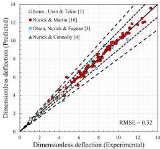
شکل (۸): مقایسه بین پیش‌بینی مدل تجربی ارائه‌شده در معادله ۱۹ و مقادیر تجربی برای بارگذاری یکنواخت
