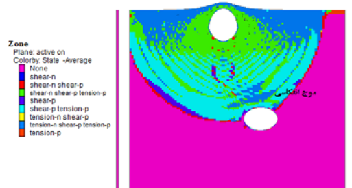
شکل (۸). حالت پلاستیک و تنش‌های اعمالی
