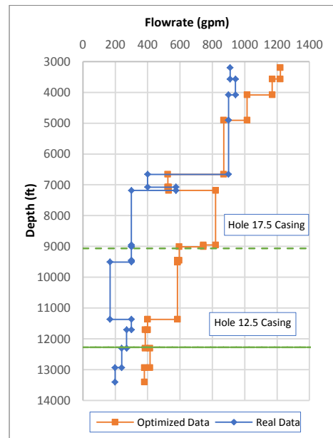
شکل (۷). مقایسه نرخ جریان سیال برای داده‌های چاه بهینه‌سازی شده و داده‌های واقعی
