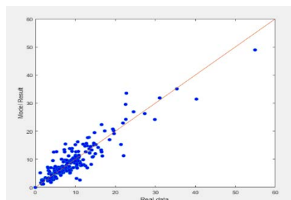
شکل (۴). مقایسه نرخ نفوذ مته واقعی و شبیه‌سازی شده توسط مدل بورگاین یانگ بهبود یافته برای تمامی حفارات.
