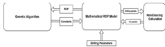
شکل (۲) فرایند مدل‌سازی عملیات حفاری
