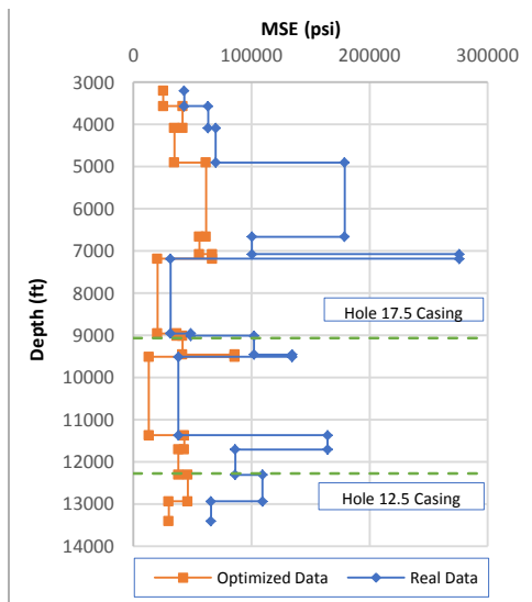
شکل (۸). مقایسه انرژی مکانیکی مخصوص برای داده‌های چاه بهینه‌سازی شده و داده‌های واقعی
