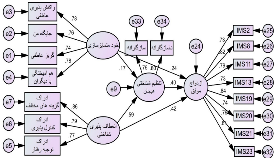
مدل ساختاری برازش شده زنان
