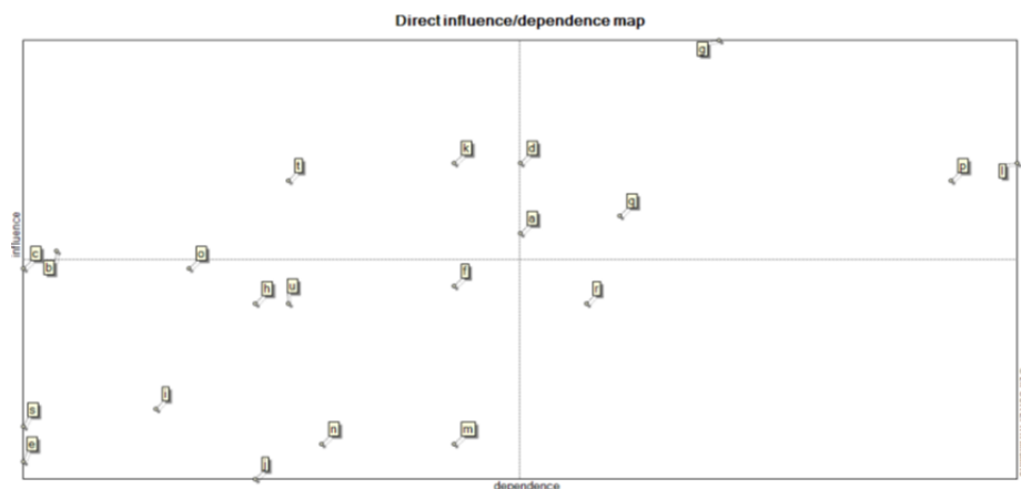
شکل ۱. نمودار اثرگذاری و اثرپذیری مستقیم عوامل بر یکدیگر
