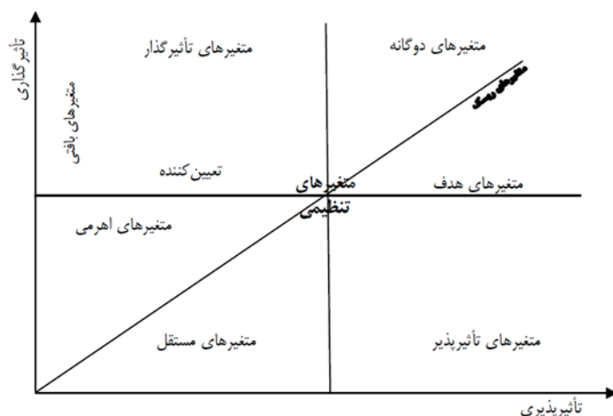
شکل ۴. الگوی توزیع انواع متغیرها در نقشه «وابستگی-تأثیر گذاری» نرم افزار میک‌مک
