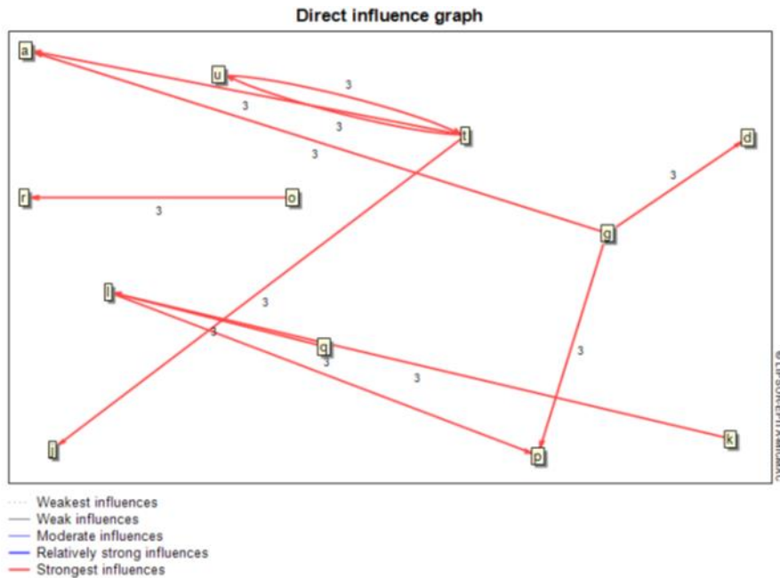
شکل ۳. تاثیرات مستقیم عوامل بر یکدیگر
