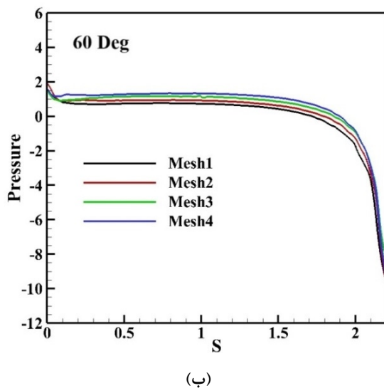
شکل (۳). تغییرات فشار روی سطح سلول سهمی شماره ۱ در زاویه ۴۵ (الف) و ۶۰ (ب) درجه به ازای ۴ شبکه‌بندی مختلف برای سرعت ۵ متر بر ثانیه
