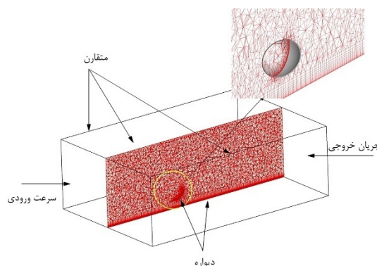
شکل (۱). هندسه مسئله، شرایط مرزی مورد نظر و شبکه محاسباتی
