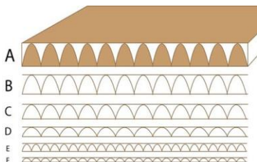
شکل (۱): انواع فلوت
