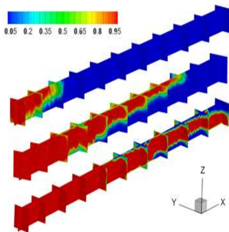
شکل (۱۴): کانتور کسر حجمی در میکرو کانال مربعی در شار گرمی 100, 300, 500 \text{ kg}/(\text{m}^2\text{s}) در قطر هیدرولیکی ۰/۷ میلی‌متر
