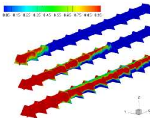
شکل (۱۱): کانتور کسر حجمی در میکرو کانال دوزنقه در شار جرمی kg/(m^2s) ۱۰۰، ۳۰۰ و ۵۰۰ در قطر هیدرولیکی 0.55 میلی متر
