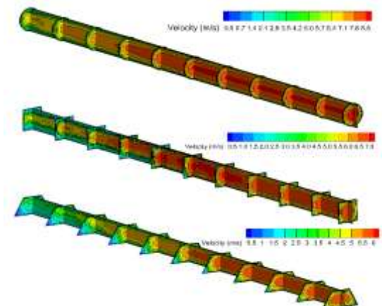
شکل (۱۸): میدان سرعت در میکرو کانالهای با مقطع دایروی، مربعی و دوزنقه با قطر هیدرولیکی ۰/۷ میلی متر و شار جرمی 400 \text{ kg}/(\text{m}^2\text{s})
