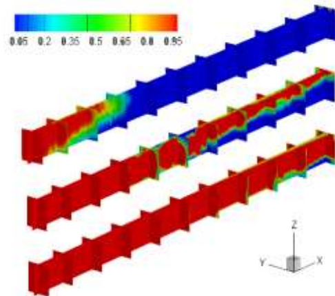
شکل (۱۳): کانتور کسر حجمی در میکرو کانال مربعی در شار گرمی 100, 300, 500 \text{ kg}/(\text{m}^2\text{s}) در قطر هیدرولیکی ۰/۵۵ میلی‌متر
