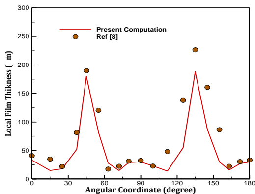
شکل (۴): مقایسه نتایج ضریب انتقال حرارت دوفاز در طول میکرو کانال با نتایج مقاله مرجع [۸]
