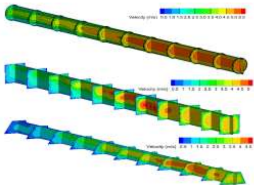
شکل (۱۷): میدان سرعت در میکرو کانالهای با مقطع دایروی، مربعی و دوزنقه با قطر هیدرولیکی ۰/۵۵ میلی متر و شار جرمی 400 \text{ kg}/(\text{m}^2\text{s})
