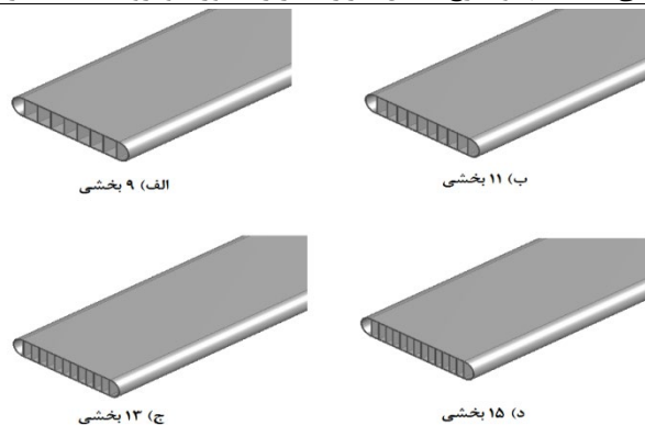
شکل (۲): شماتیک لوله دارای ریز مجرا
