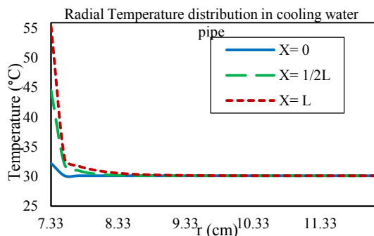
شکل (۳): توزیع شعاعی دمای آب سرد در پوسته بیرونی در سه مقطع از مبدل حرارتی دو لوله‌ای
