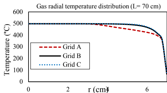
شکل (۲): توزیع شعاعی دمای دود در خروجی مبدل حرارتی دو لوله‌ای برای سه شبکه بررسی شده
