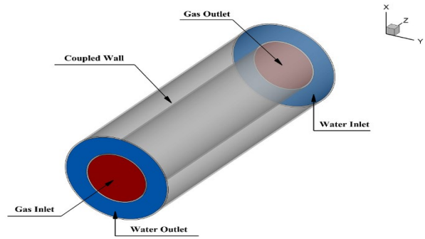
شکل (۱): شرایط مرزی مبدل حرارتی دو لوله‌ای
