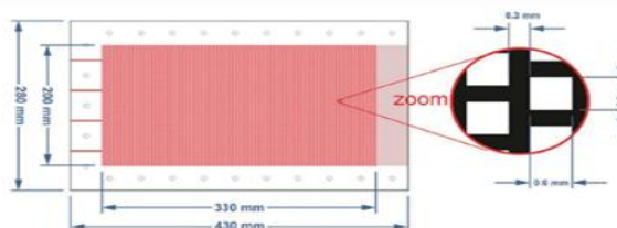
شکل ۲. طراحی محیط متخلخل مورد استفاده در پژوهش
