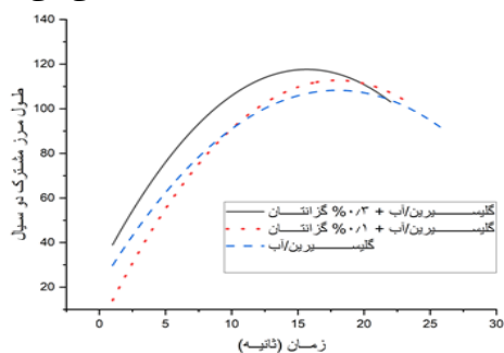
شکل ۶. تغییرات پارامتر طول مرز مشترک با گذشت زمان در طول سلول برای سیالات مختلف پر شده محیط متخلخل
