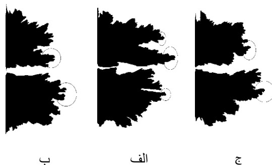
شکل ۸. پیشروی انگشتی غالب تولید شده در محیط متخلخل در ثانیه ششم تزریق برای سیال بستر الف) گلیسیرین / آب ب) گلیسیرین / آب + ۰,۱٪ گزانتان گام ج) گلیسیرین / آب + ۰,۳٪ گزانتان گام
