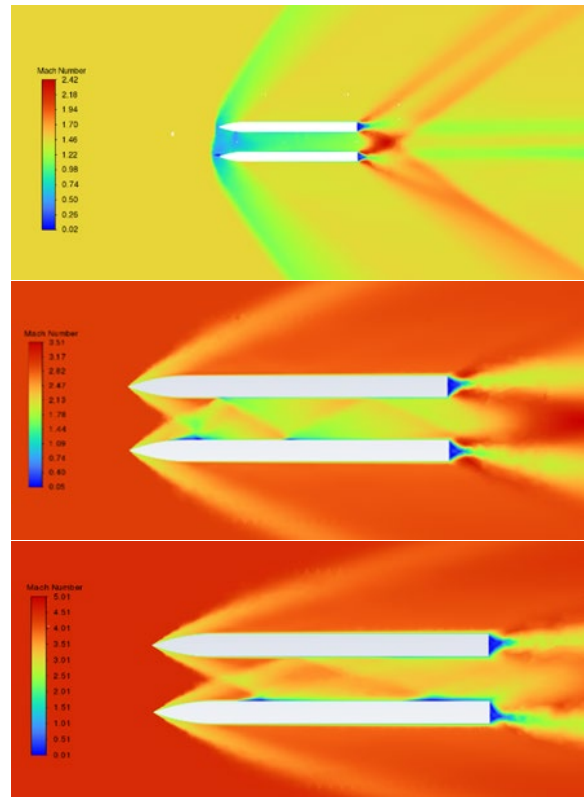
شکل (۱۴): کانتور سرعت در حالت دارای حرکت نسبی دوبدنه باریک دوبعدی در سرعت جریان آزاد ۱/۵ (بالا)، ۳ (وسط) و ۴/۵ (پایین) ماخ در حالت سه‌بعدی با فاصله محورهای سه برابر قطر بدنه باریک.
