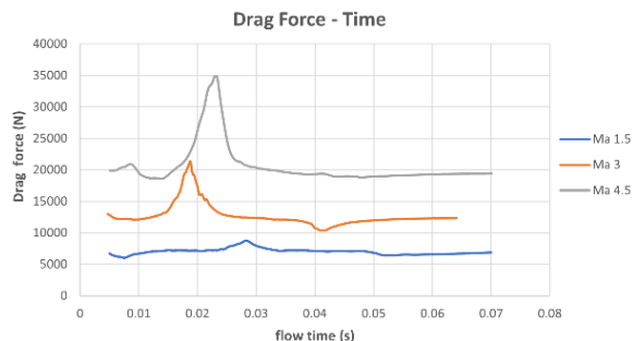
شکل (۲۷): نیروی درگ بر روی بدنه باریک پایینی در حین عبور از نزدیکی بدنه باریک بالایی در فاصله بین محورهای 3 برابر قطر هر کدام و سرعت جریان آزاد 1/5 ، 3 و 4/5 ماخ.
