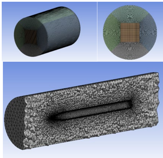
شکل (۵): شبکه مستقل سه‌بعدی، شامل مش زمینه (سازمان‌یافته) و مش اطراف بدنه باریک (بی‌سازمان).
