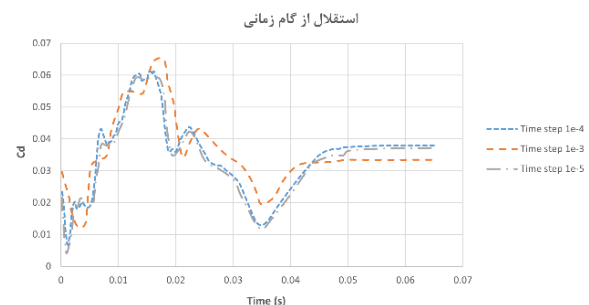
شکل (۶): روند استقلال از گام زمانی با در نظر گرفتن ضریب درگ در بازه زمانی ۰/۰۷ ثانیه.
