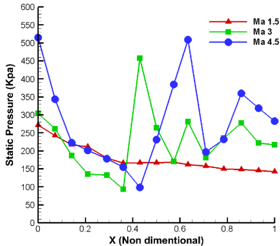
شکل (۱۶): تغییرات فشار استاتیکی در طول بدنه باریک پایینی در حالت بدون حرکت نسبی و دوبعدی در فاصله بین محورهای ۳ برابر قطر بدنه باریک.
