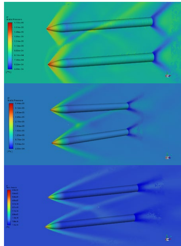
شکل (۲۲): کانتور تغییرات فشار استاتیکی در طول بدنه باریک پایینی در حالت سه‌بعدی دارای حرکت نسبی در فاصله بین محورهای ۳ برابر قطر بدنه باریک در ماخ جریان آزاد ۱/۵ (بالا)، ۳ (وسط) و ۴/۵ (پایین).
