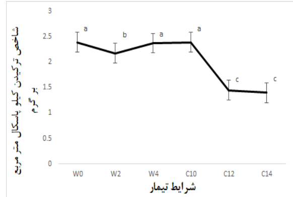
شکل (۶): مقایسه میانگین شاخص مقاومت در برابر ترک‌شدن کاغذهای مختلف
