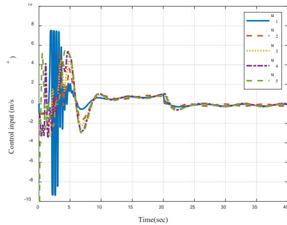
شکل (۹): ورودی کنترلی خودروهای پیرو در سناریوی
