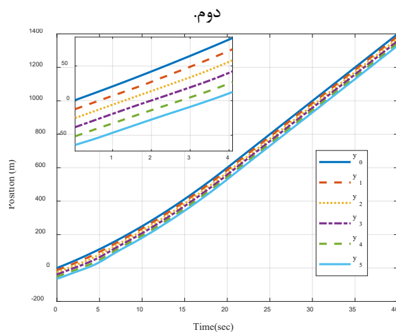
شکل (۱۰): موقعیت خودروهای پیرو در سناریوی دوم.
