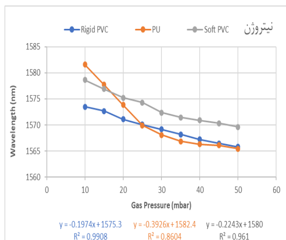
شکل (۹). نمودار تغییرات طول موج بر حسب فشار گاز نیتروژن برای تمامی حسگرها
