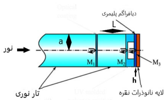
شکل (۱). طرح‌واره حسگر فیبر نوری فابری-پرو دیافراگمی
