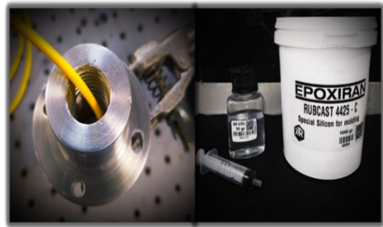
شکل (۳). قرارگیری حسگر در قطعه آلومینیومی و ریختن اپوکسی درون آن
