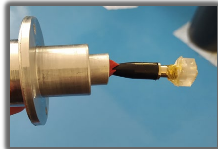
شکل (۴). حسگر فیبر نوری فابری-پرو با لایه PU
