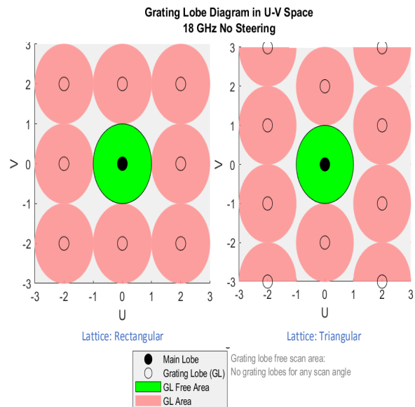
شکل ۴- منطقه‌ی اسکن بدون حضور گریتینگ لوب
