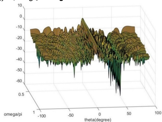
شکل ۱۶- شکل دهی پرتو برای فراست با اسنپ‌شات بالا، N_h = 10000
