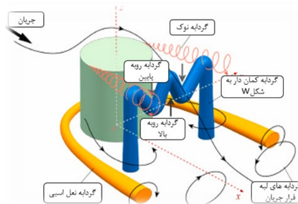
شکل (۱): فیزیک جریان حول استوانه محدود [۹]
