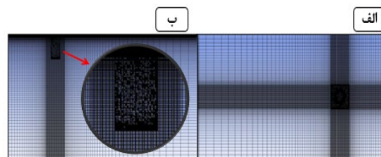
شکل (۵): (الف) نمای فوقانی شبکه‌بندی در هندسه سه‌بعدی (ب) نمای جانبی شبکه‌بندی در هندسه سه‌بعدی
