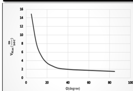
شکل (۹): محدوده اندازه‌گیری سرعت بر حسب زاویه
