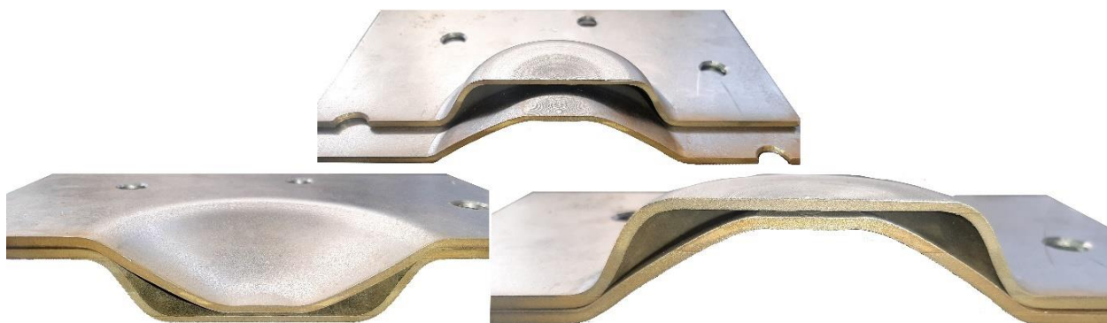
شکل (۱۳): نمای برش خورده و داخلی نمونه ورق‌های تغییر شکل یافته در فرآیند شکل‌دهی انفجاری زیر آب با قالب مادگی بدون راهگاه.
