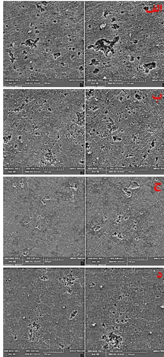
شکل (۱۱): تصاویر میکروسکوپ الکترونی روبشی از سطح خوردگی نمونه‌های آلومینیوم آلیاژی ۶۰۶۱ فرآوری شده با فرایند پرس کاری شیپارمقید: (الف) نمونه اولیه آنیل شده، (ب) نمونه تک پاسه، (ج) نمونه دو پاسه و (د) نمونه چهار پاسه.
