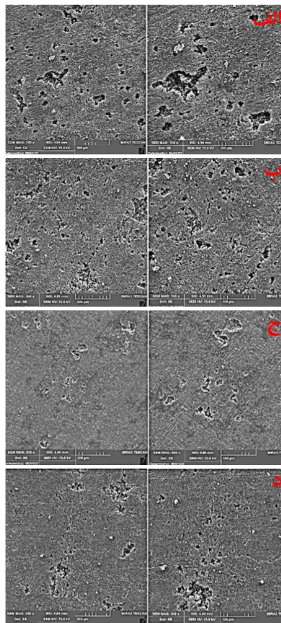
شکل (۱۱): تصاویر میکروسکوپ الکترونی روبشی از سطح خوردگی نمونه‌های آلومینیوم آلیاژی ۶۰۶۱ فراوری شده با فرایند پرس کاری شیارمقید: (الف) نمونه اولیه آنیل شده، (ب) نمونه تک پاسه، (ج) نمونه دو پاسه و (د) نمونه چهار پاسه.
