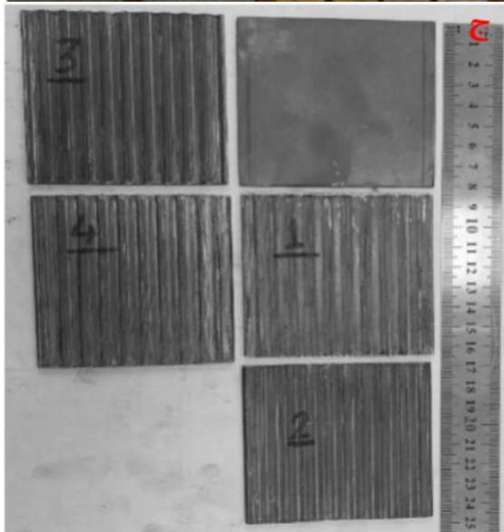
شکل (۳): نحوه فراوری نمونه‌های آلومینیوم آلیاژی ۶۰۶۱:
