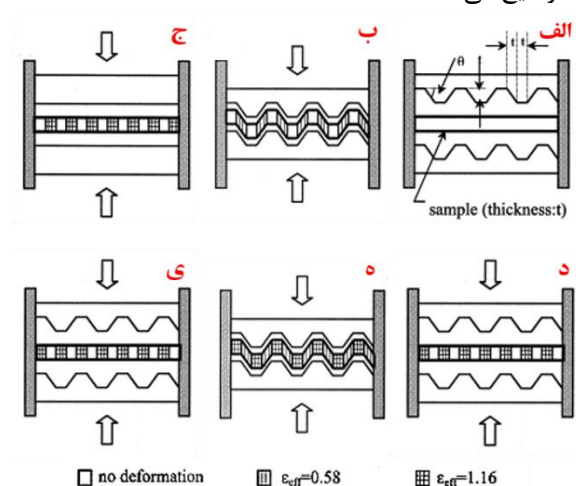
شکل (۱): طرحواره مراحل مختلف انجام فرایند پرس کاری شیارمقید در طول یک پاس [۱].
