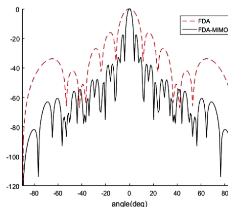
شکل (۷). مقایسه پترن FDA و FDA-MIMO خطی
