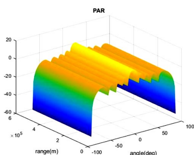
شکل (۴). الگوی پرتو در رادار آرایه متغیر فرکانسی بدون افزایش فرکانس \Delta f = 0 ، PAR
