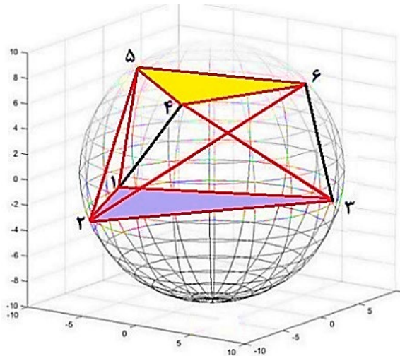
شکل (۶): تنسگریتی منشوری با شش گره و محاط بر کره.
