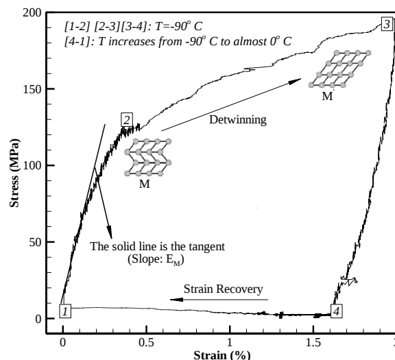
شکل (۹): نمودار تنش-کرنش و فرایند غیر دوقلویی یا تک واریانت شدن سیم SMA نایتینول غنی از نیکل در حالت مارتنیزیت کامل ( -90^{\circ}\text{C} ) به همراه رفتار شبه‌پلاستیک و بازیابی کرنش در نتیجه گرما دادن تا حصول دمایی بالاتر از دمایی پایان آستنیت ( A_f ).
