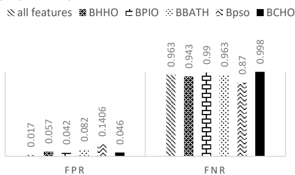
شکل (6): مقایسه معیارهای ارزیابی بر روی سه مجموعه داده
