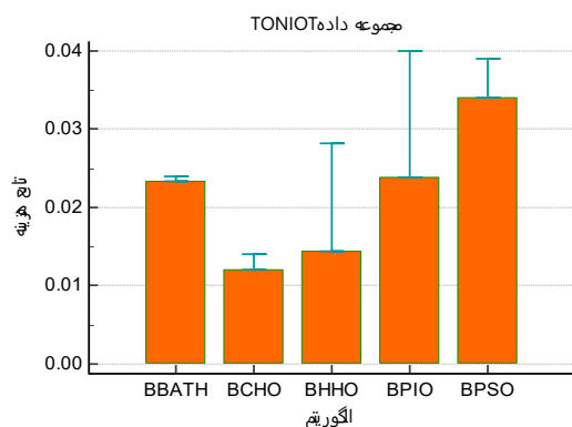
شکل (8): نتایج آزمون کروسکال-والیس بر روی مجموعه داده TON-IOT
