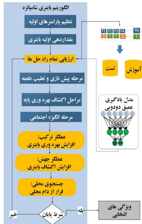
شکل (2): فلوچارت روش پیشنهادی انتخاب ویژگی BCHO
