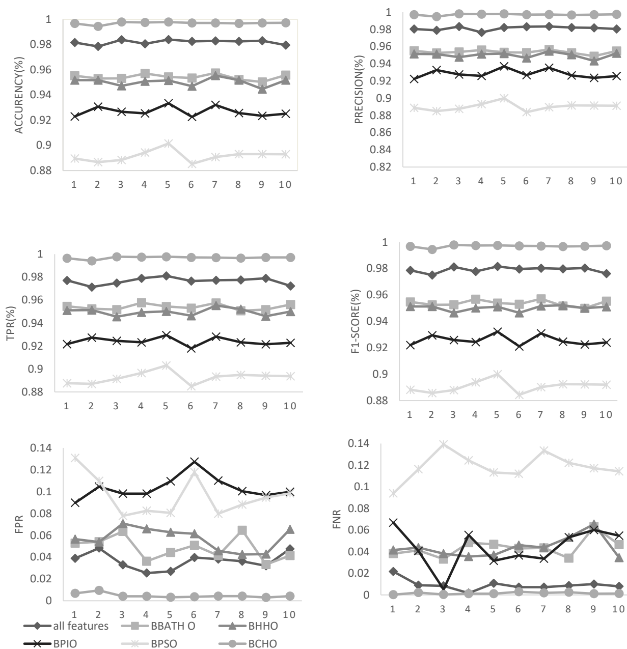
شکل (4) نتیجه K-FOLD بر روی مجموعه داده UNSWNB15
