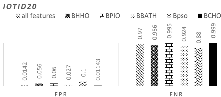
شکل (7): مقایسه معیارهای FPR, FNR بر روی سه مجموعه داده
