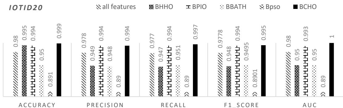
شکل (6): مقایسه معیارهای ارزیابی بر روی سه مجموعه داده
