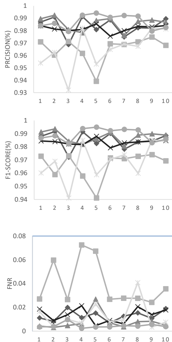
شکل (3) نتیجه K-FOLD بر روی مجموعه داده TONIOT
